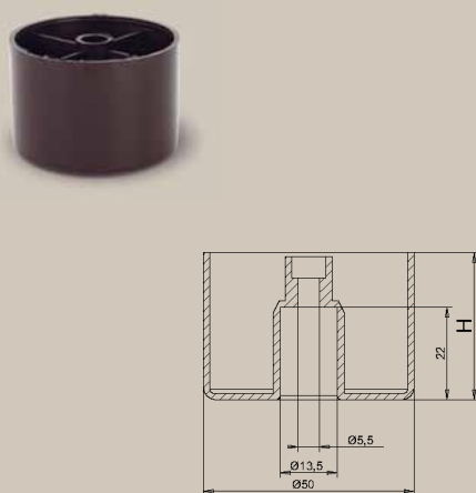
TS 026-5 H=65 TS 129-5 H=100
