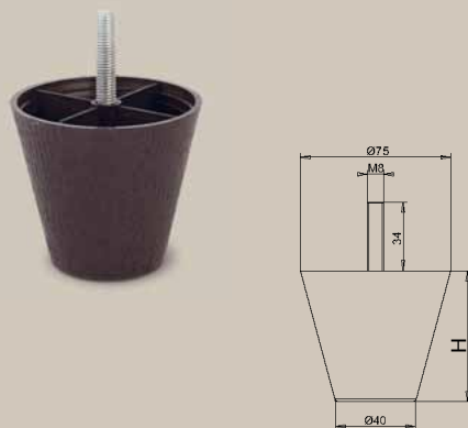
TS 026-5 H=65 TS 129-5 H=100
