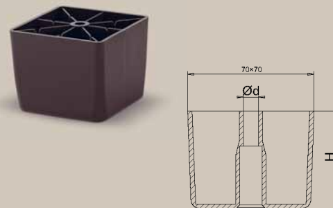
TS 063-5 H=55 Ød=8,5 TS 184-5 H=45 Ød=7
